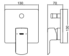
TBN01001B Concealed Box Mini Unit
